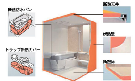
断熱材パック・断熱防水パン
